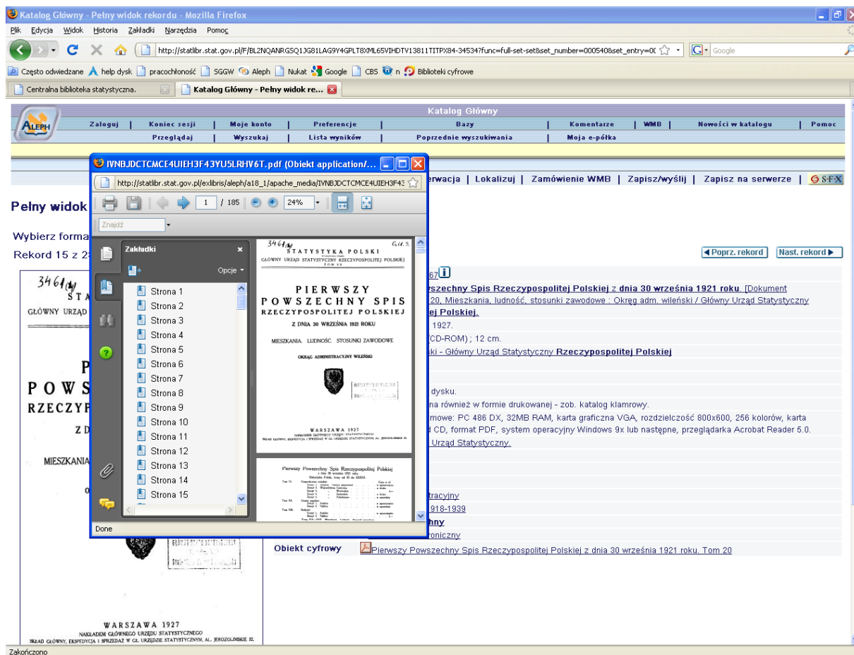
Rys.11 Publikacja otwieranie
