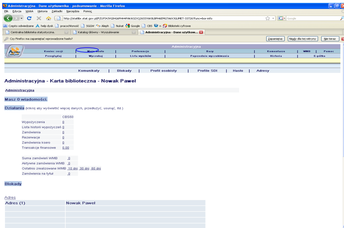
Rys.6 Moje konto
